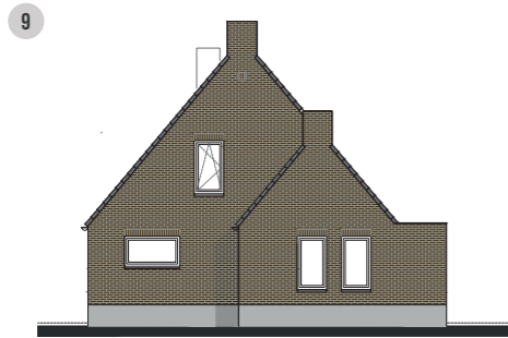
Rechtergevel Tweekappers
