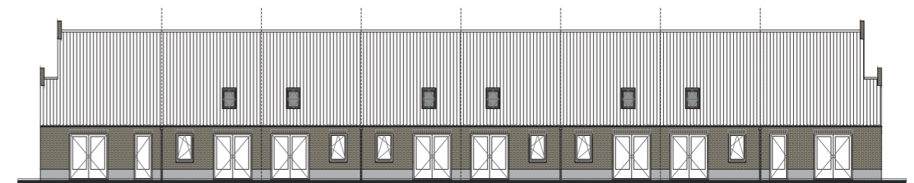
NOORDWEST-GEVEL
